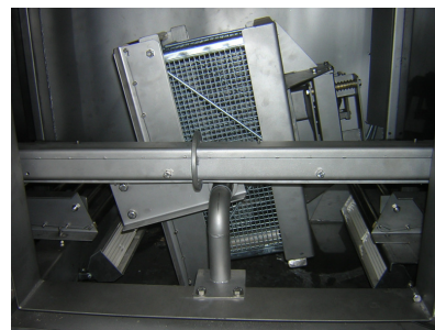
Rotation av korg i vätsteg och tork. Vinkel och hastighet är steglöst justerbart.
